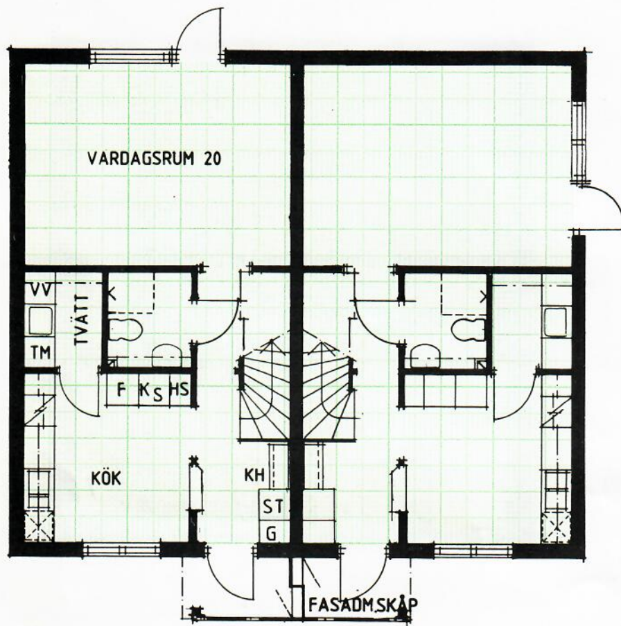
BOTTENVÅNING
