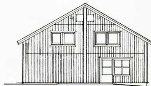
TRÄDGÅRDSFASAD
