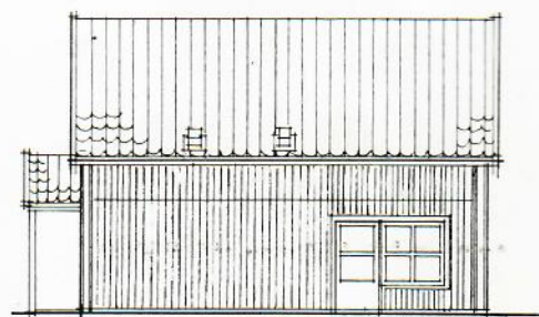
LÅNGFASAD HÖGER
