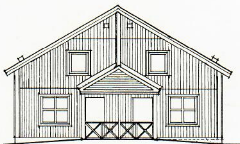
ENTREFASAD
